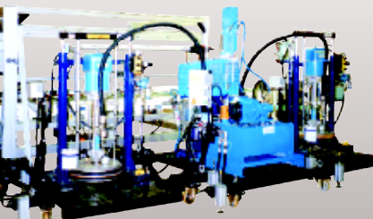
COLLAGE DES PANNEAUX D'ÉTANCHÉITÉ à l'intérieur des méthaniers
